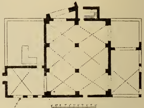
10654. — Plan de la maison d'Equitius dans son état primitif.
